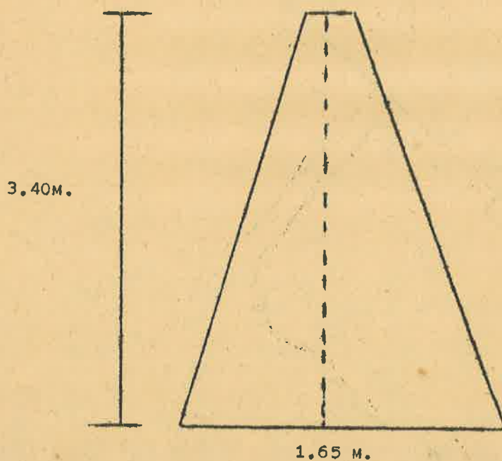
CORTE DEL MURO EXTERNO
