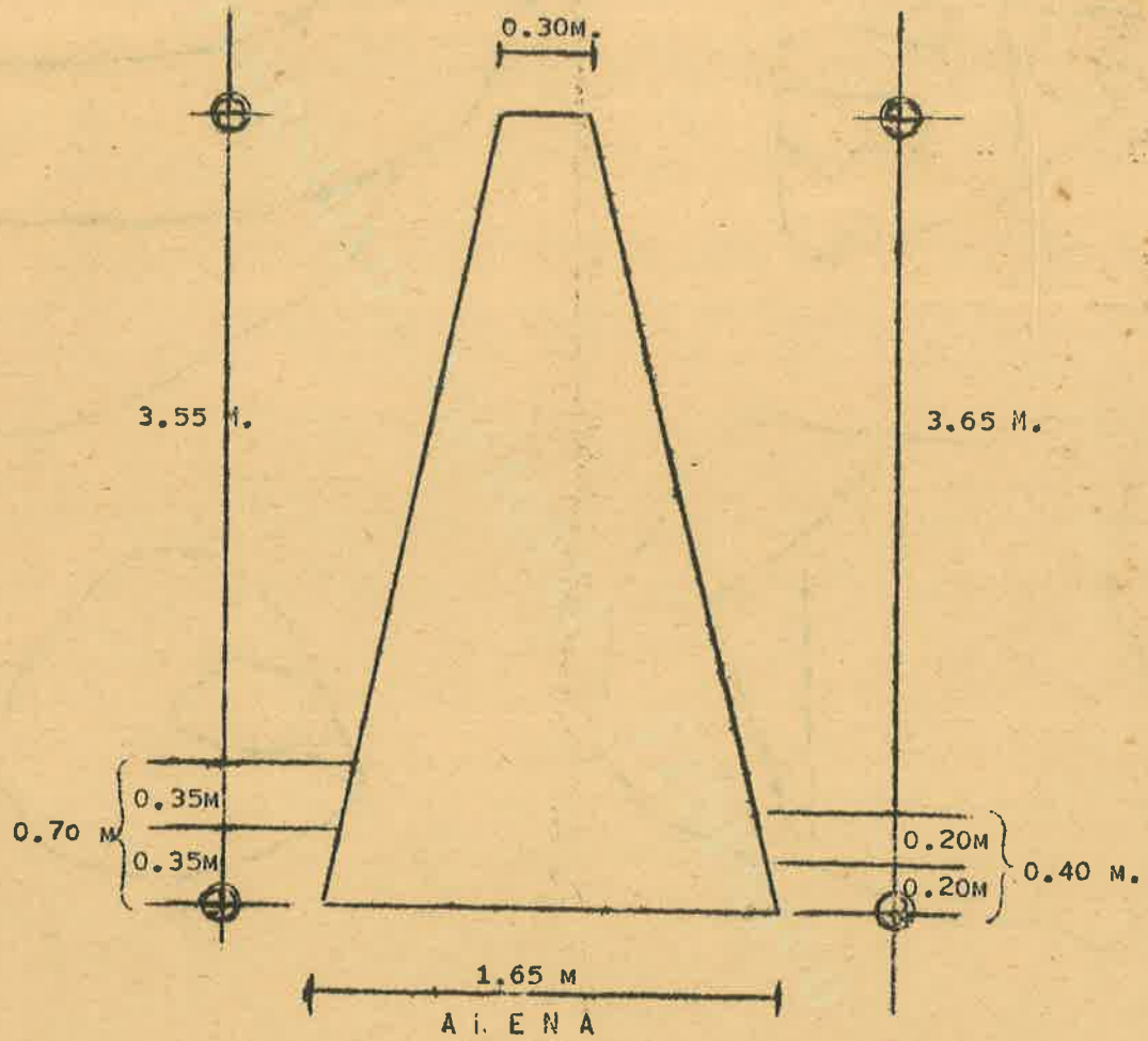
CORTE DEL MURO EXTERNO EN FORMA TRIANGULAR
